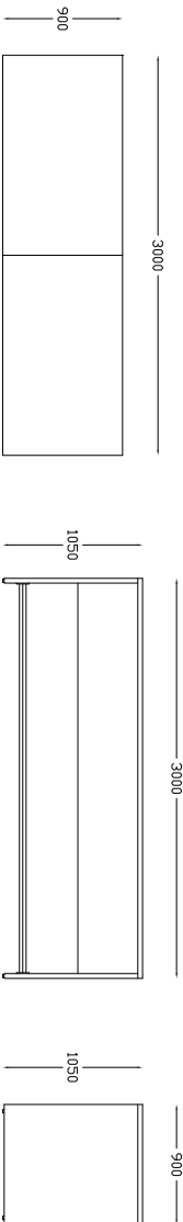
W 2700 X D 900 X H 1050
